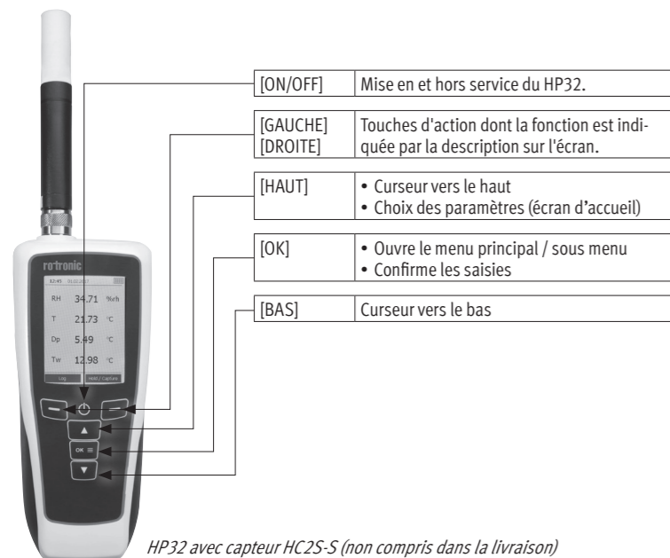
HP32 avec capteur HC2S-S (non compris dans la livraison)
